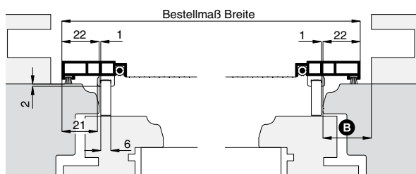
Horizontalschnitt
