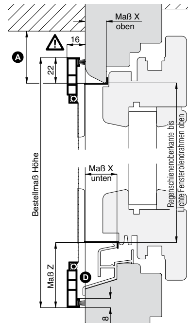
Vertikalschnitt
