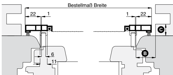
Horizontalschnitt
