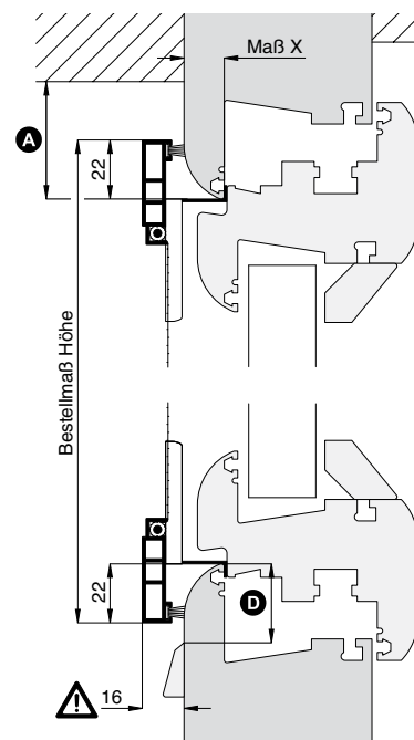
Vertikalschnitt
