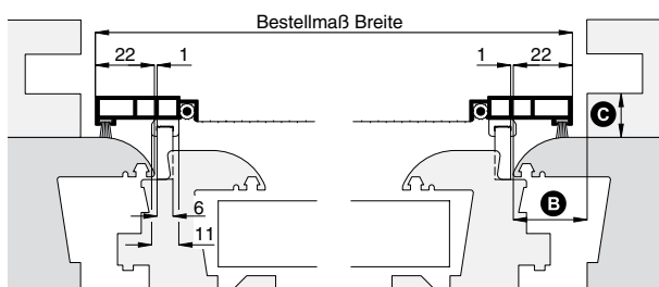
Horizontalschnitt
