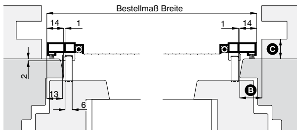
Horizontalschnitt
