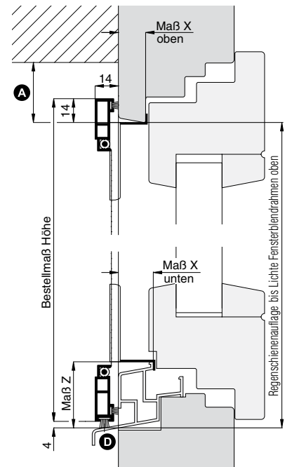
Vertikalschnitt
