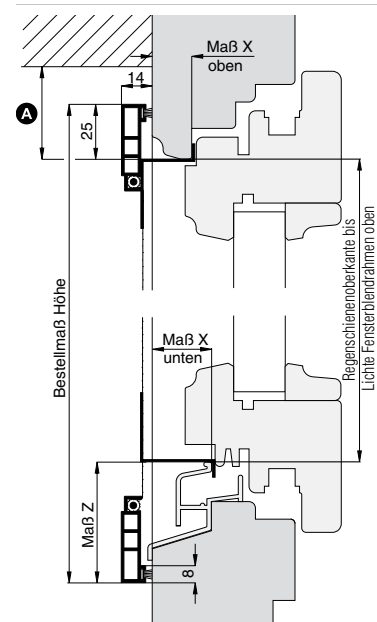
Vertikalschnitt
