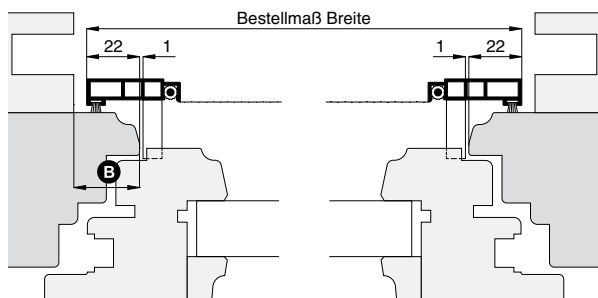
Horizontalschnitt
